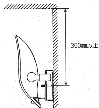
天井からの取付距離
