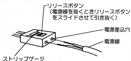
図-1 SL端子台
