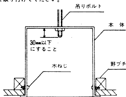
吊りボルトまたは木ねじによる固定
