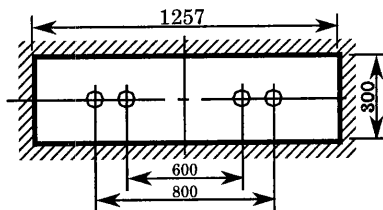
単体取付
