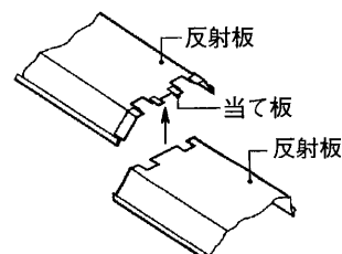
連結用器具の場合
