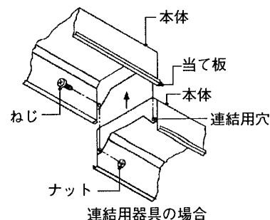
連結用器具の場合
