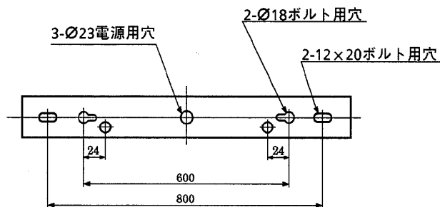
背面仕様図
