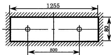
単体取付
