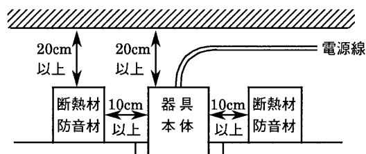
連結取付
