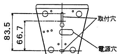
器具取付寸法図
