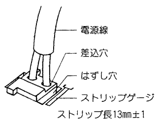
図-1 電源線接続方法
