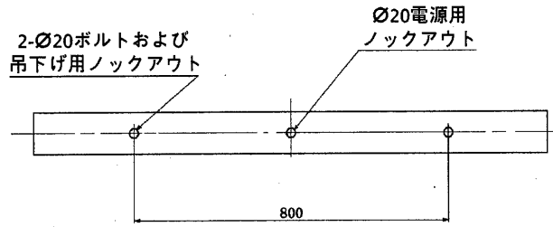
背面仕様図
