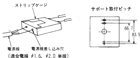
図2 SL端子台
