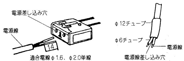
図-1 SL端子台 保護チューブの取り付け方
