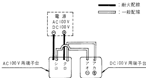
※2線引配線の場合
