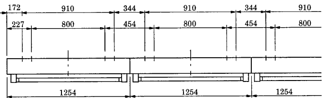
連結寸法図
