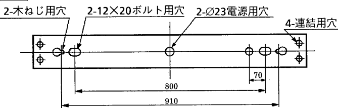
背面仕様図
