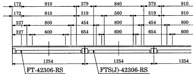
連結寸法図
