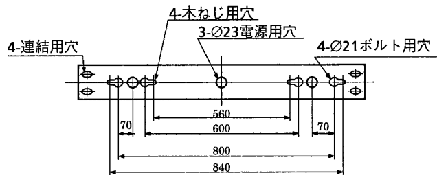
背面仕様図
