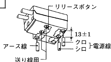
電源端子台
