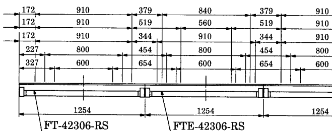
連結寸法図
