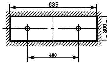
単体取付
