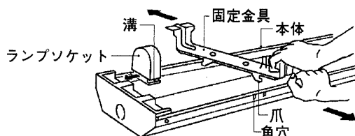
連結取付
