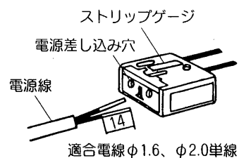
図-2 SL端子台
