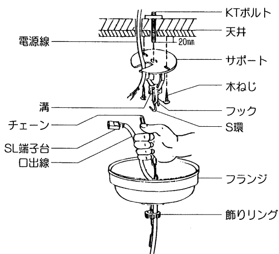
図-1 SL端子台
