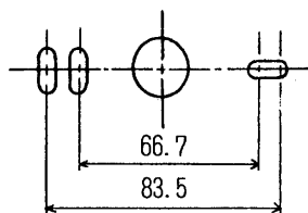
本体取付ピッチ
