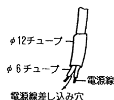
保護チューブの取り付け方
