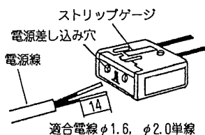
図-2 SL端子台
