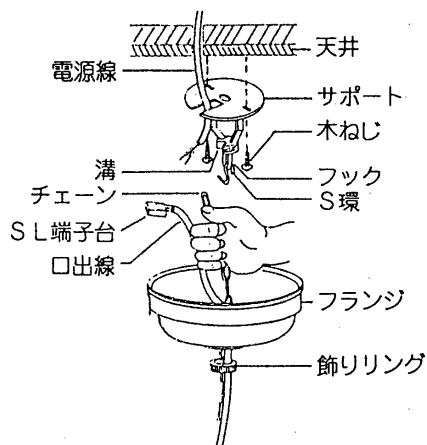
図-2 SL端子台
