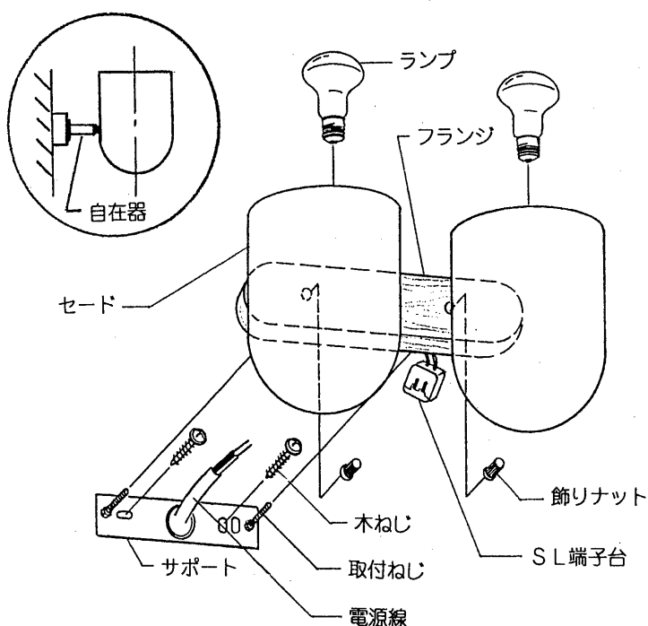
図-1 SL端子台
