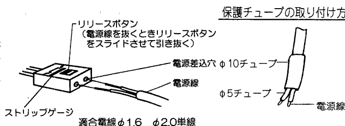
図-1 SL端子台
