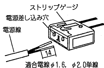
図-1 SL端子台
