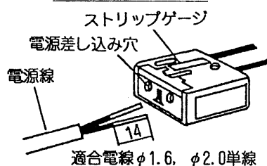
図-3 SL端子台
