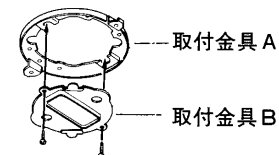
角形引掛シーリング
