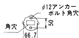
取付金具B
