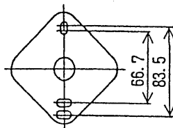
サポートの取付ピッチ
