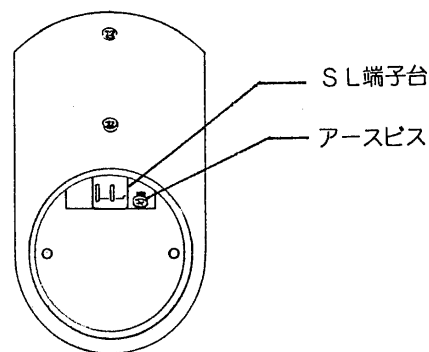
図-2 陶器本体の内面
