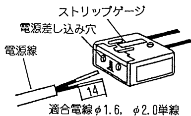
図-1 SL端子台
