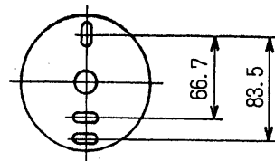
サポート取付ピッチ
