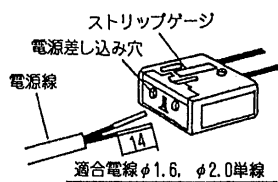
図-2 SL端子台
