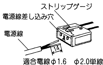
図-2 SL端子台
