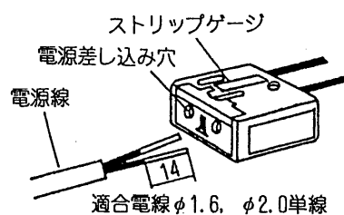
図-2 S L 端子台
