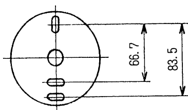
サポート取付ピッチ
