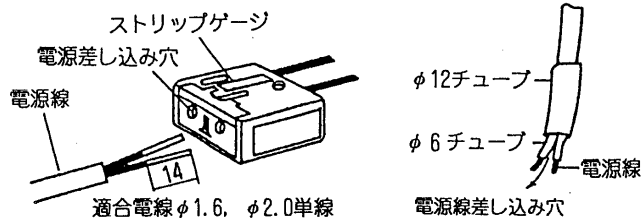
図-1 SL端子台
