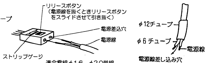
図-1 SL端子台
