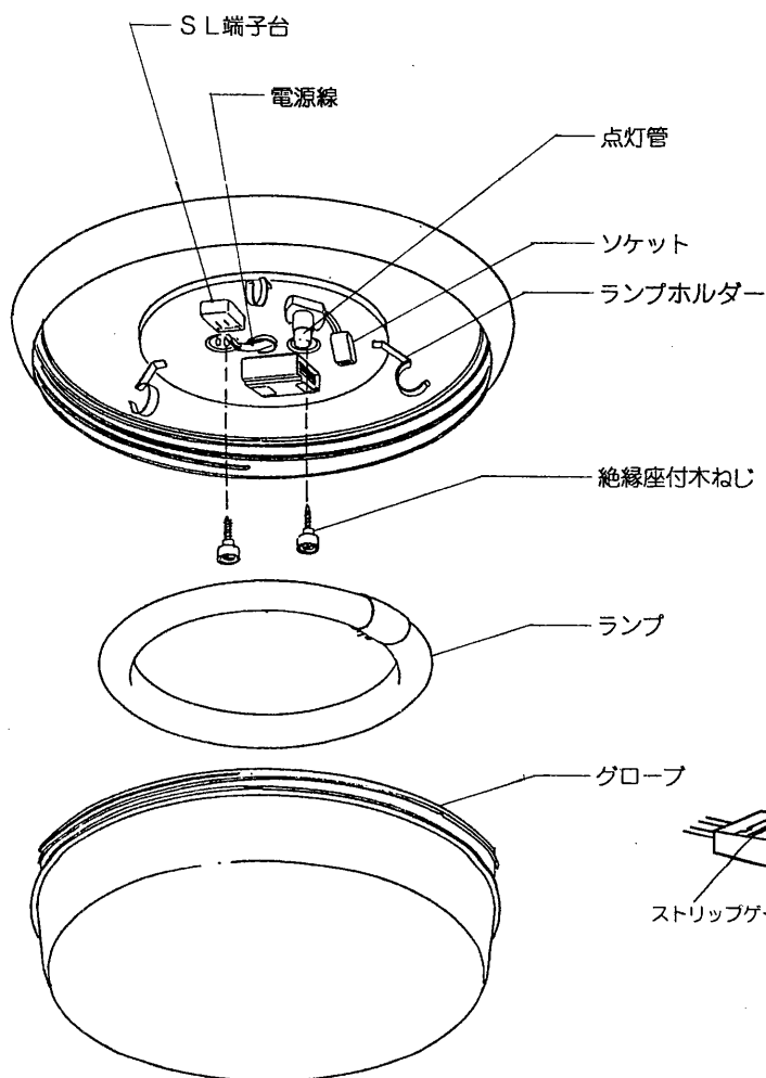
図-1 SL端子台
