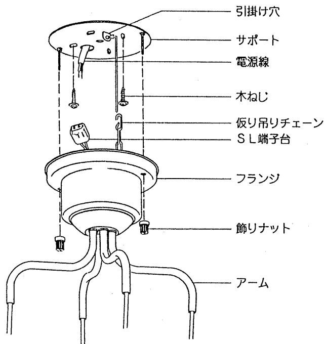
図-1 SL端子台
