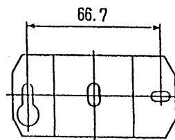
サポートの取付ピッチ
