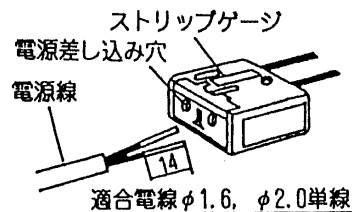
(図-1) SL端子台
