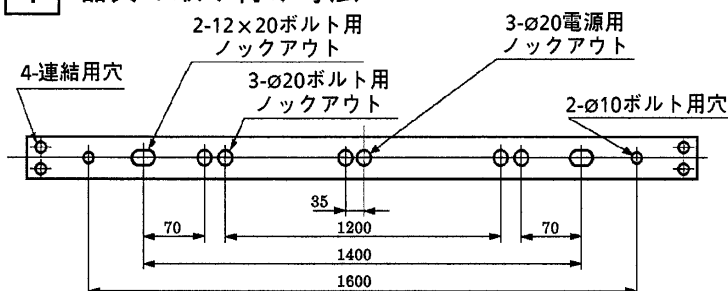
背面仕様図
