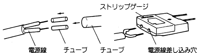
図 2 SL 端子台
