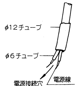
保護チューブ取り付け方
