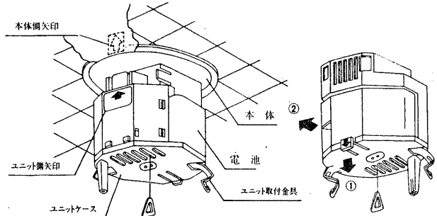
〔図5〕 ユニットの取り付けかた
