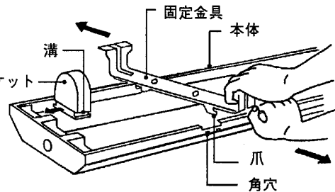
連結取付
