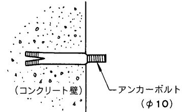
取付寸法図
