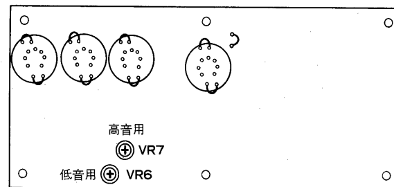
マッチングトランス取付用基板(P-486-012A)
