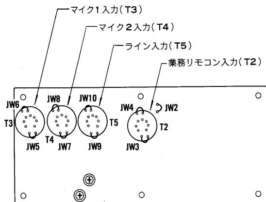
マッチングトランス取付用基板 (P-486-012A)
