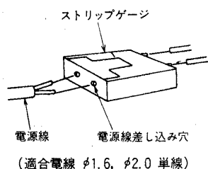
図2 SL端子台
