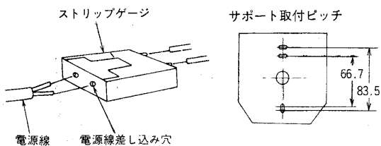
図2 SL端子台
