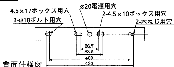
背面仕様図
