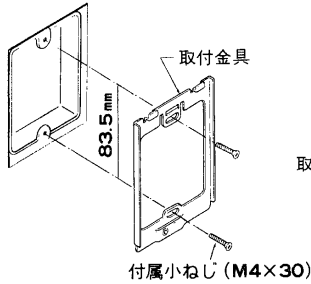
付属小ねじ (M4×30)
