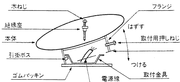
図2 端子接続は確実にこなして下さい
