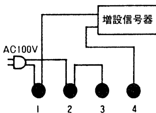
●AC100V器具の場合
