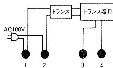
●トランス器具の場合
