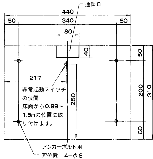
取付寸法図
