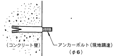
取付寸法図
