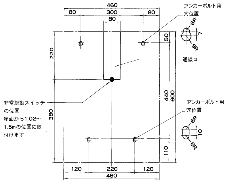
取付寸法図
