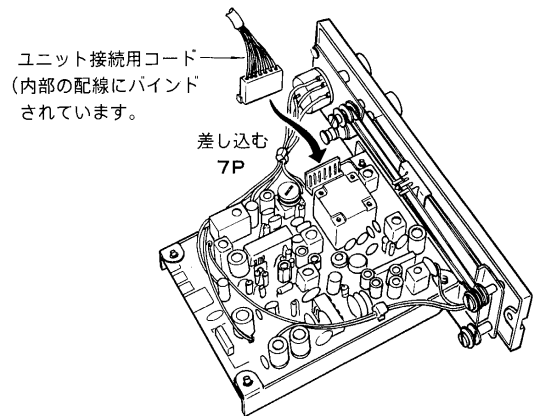
ユニット（別売） （ARU-2100A, ARU-2100AF） （ARU-2200AF, ATU-1100C）
