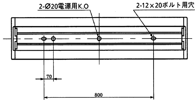
背面仕様図
